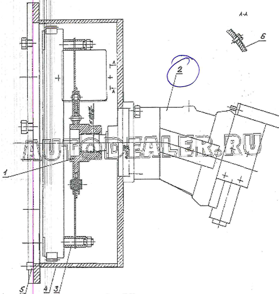
Рис. 43 Установка насоса
